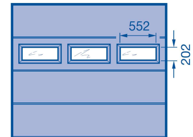
Mit Kassettenfenster M0
